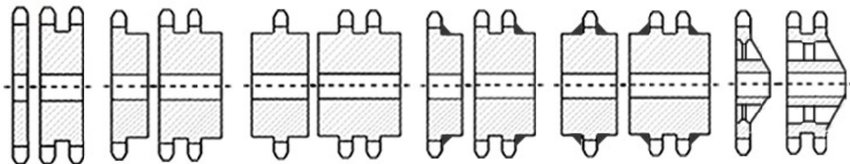
Tipo 1 totalmente usinada Tipo 2 totalmente usinada Tipo 3 totalmente usinada Tipo 4 cubo soldado Tipo 5 cubos soldados Tipo 6 totalmente usinada
